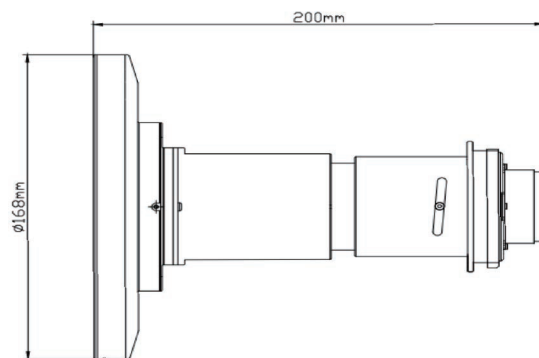
外形尺寸圖
