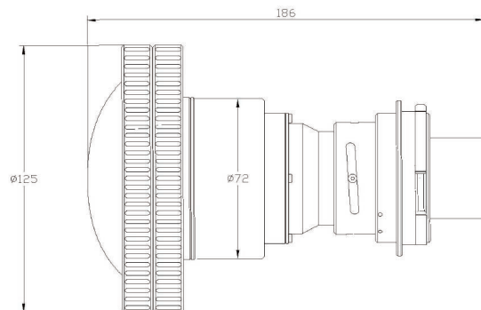
外形尺寸圖
