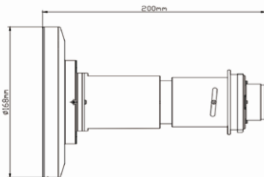
外形尺寸圖
