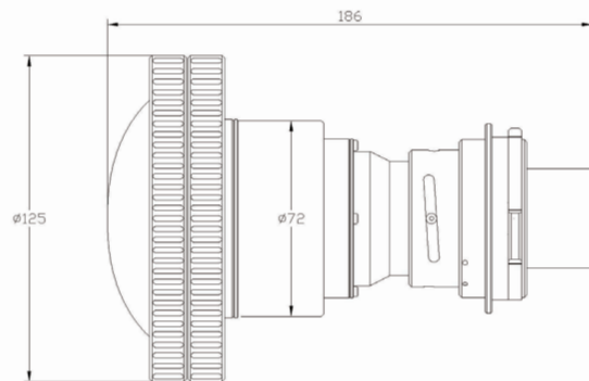
外形尺寸圖
